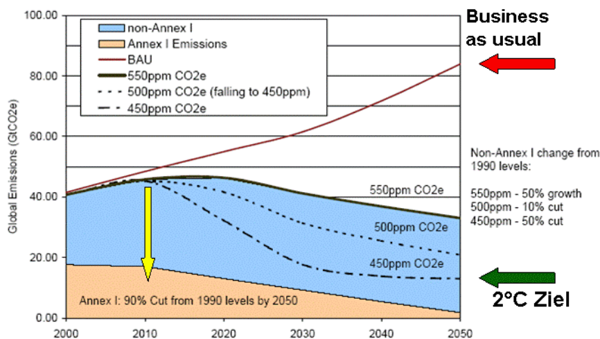
Abbildung 3-3: Erforderliche THG-Emissionsreduktionen zur Stabilisierung des Klimawandels [Stern 2006; verändert]
