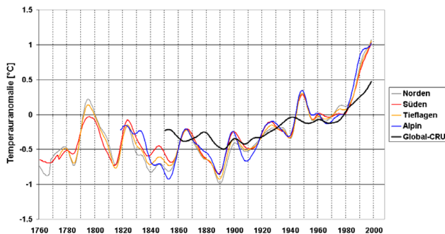
Abbildung 3-1: Temperaturverlauf im Alpinen Raum und im globalen Mittel (Datenquelle: ZAMG)
