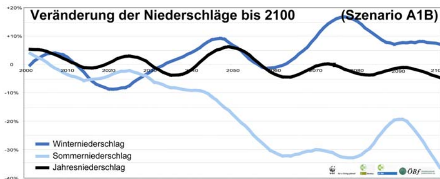
Abbildung 4-4: Entwicklung der Jahresniederschläge in Österreich nach dem A1B Szenario bis Ende 2100. (Niedermair et al., 2007)
