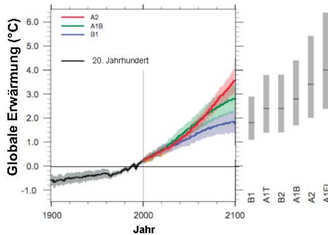
Abbildung 3-2: Temperaturanstieg bis zum Ende dieses Jahrhunderts für verschiedene Szenarien nach IPCC 2007
