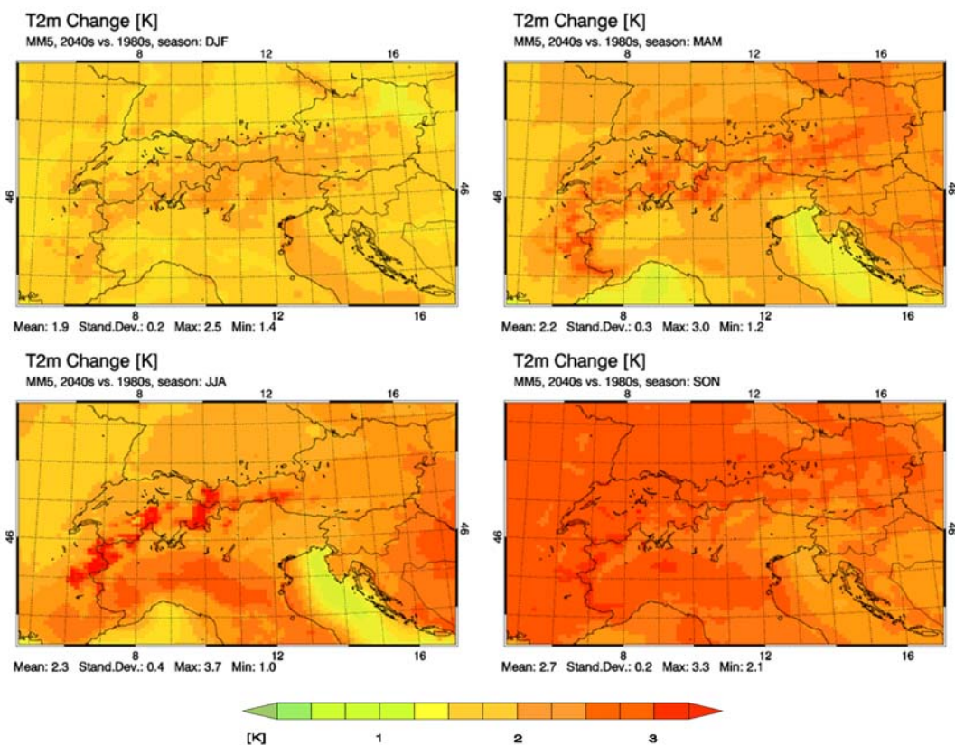
Abbildung 4-1: Änderung des saisonalen Temperaturdurchschnitts (T2m) in °C für 2041-2050 im Vergleich zu 1981- 1990. Dargestellt für das Regionalmodell MM5. (Loibl et al., 2007)
