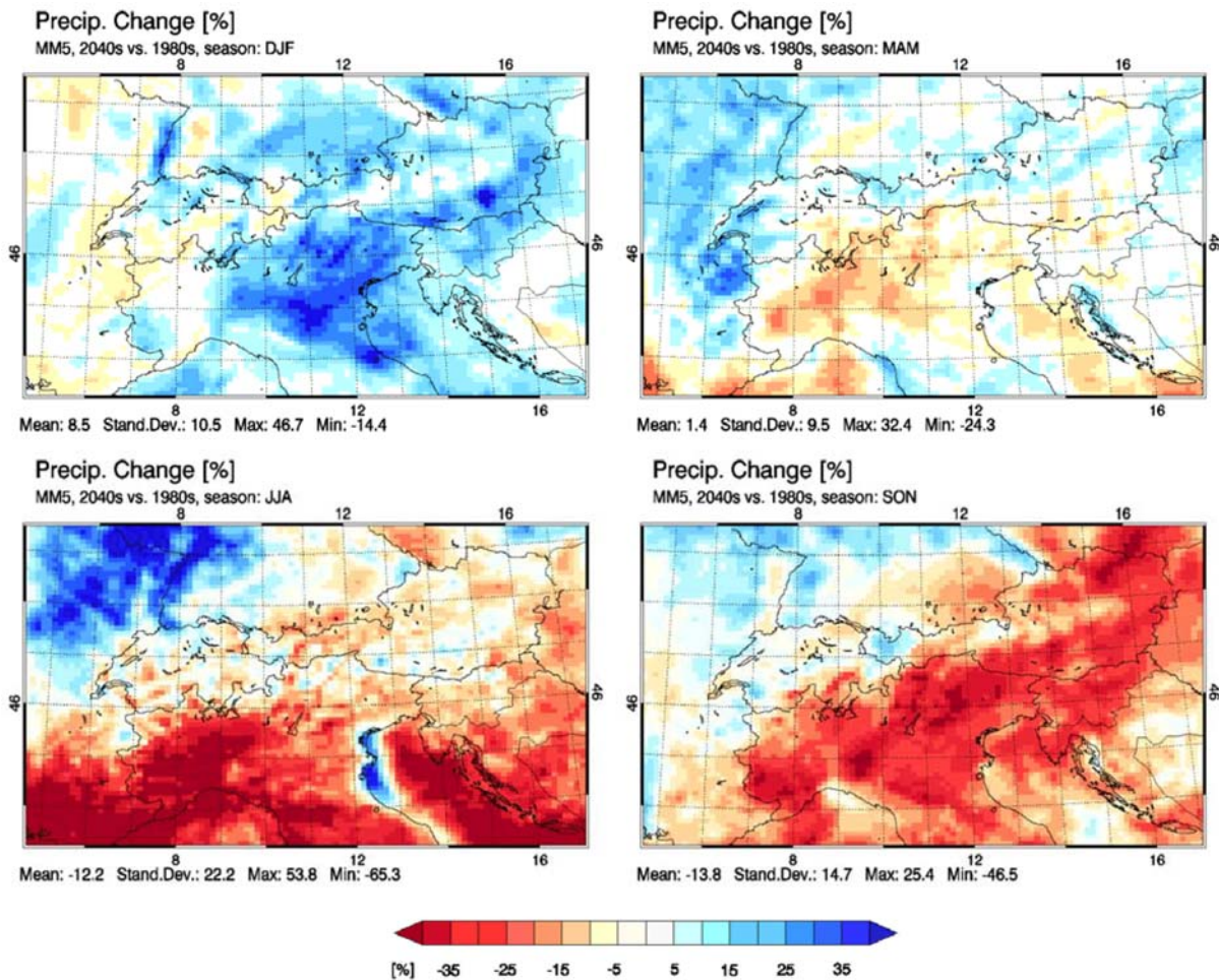
Abbildung 4-3: Änderung des saisonalen Niederschlages in Prozent für 2041-2050 im Vergleich zu 1981-1990. Dargestellt für das Regionalmodell MM5. (Loibl et al., 2007)
